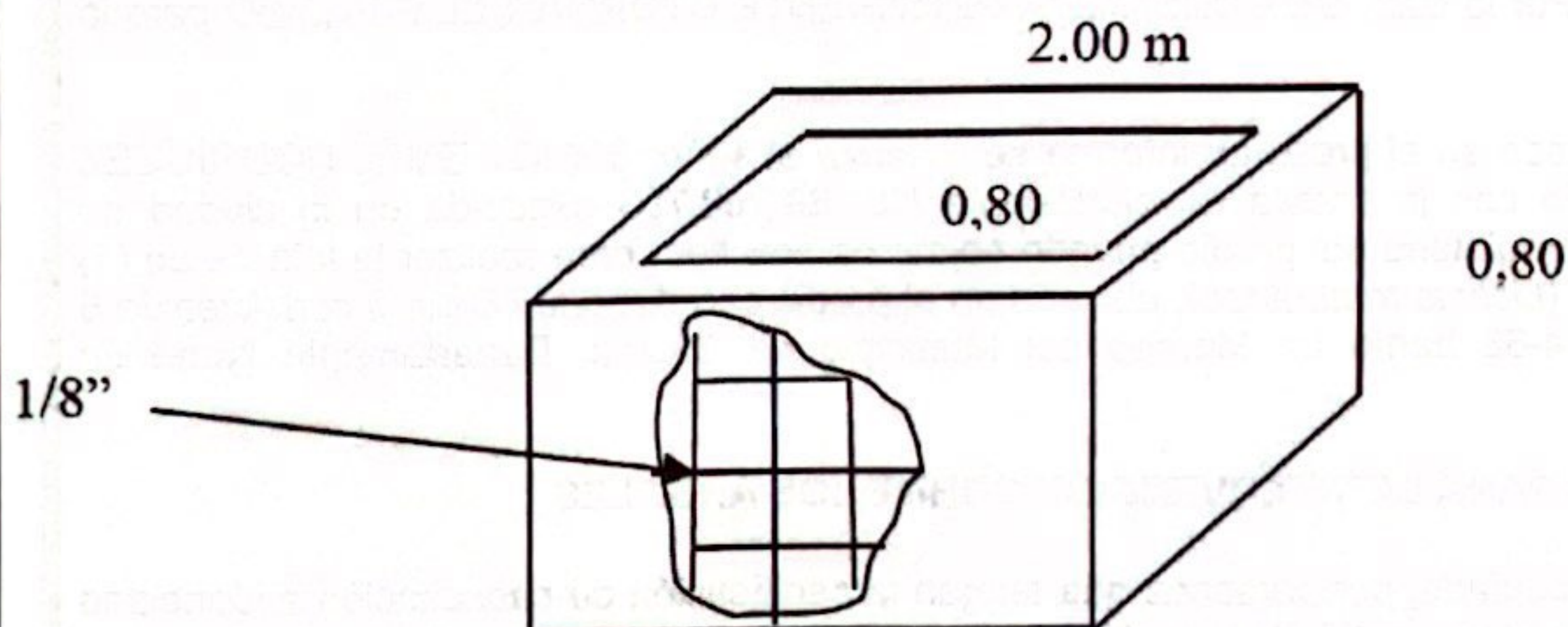
Estructura en concreto reforzado con dimensiones externas de 1,00 metros x 2,00 metros por lado y 0,60 cms de largo Con refuerzos de 1/8" y concreto 1:2:3.
