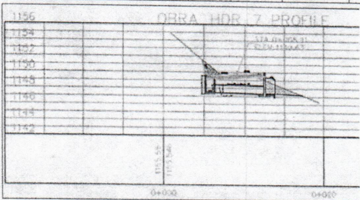
Imagen 6. Perfil Estructura Hidráulica 7
